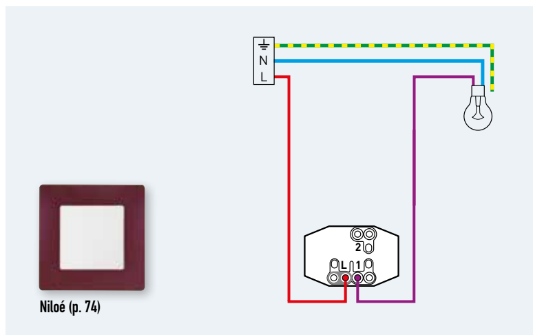
1 punto de luz (interruptor)
