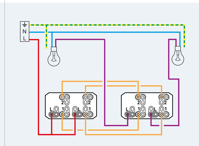
2 módulos de mando por lámpara (conmutador)
