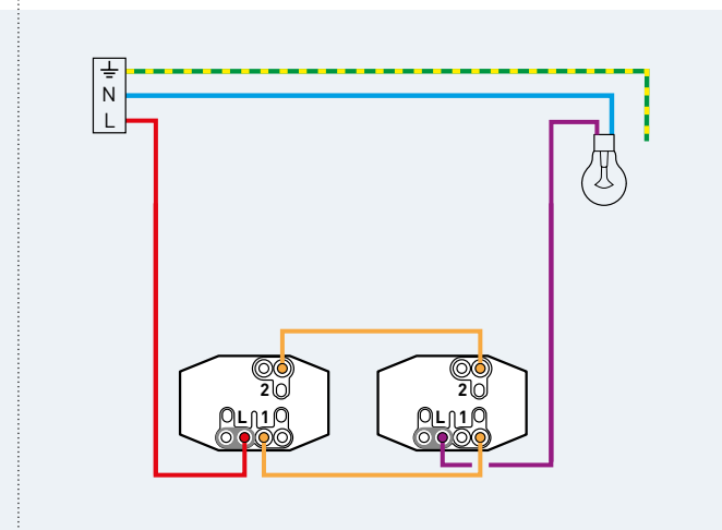
2 puntos de luz (conmutador)
