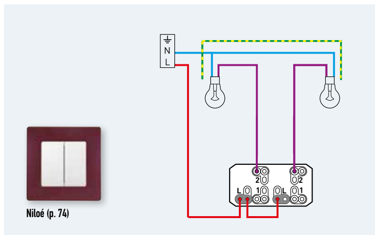
1 módulo de mando por lámpara (interruptor)
